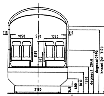
Doorsnede Coupe AA
